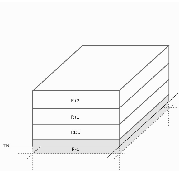
Figure 16 : Niveau semi-enterré
